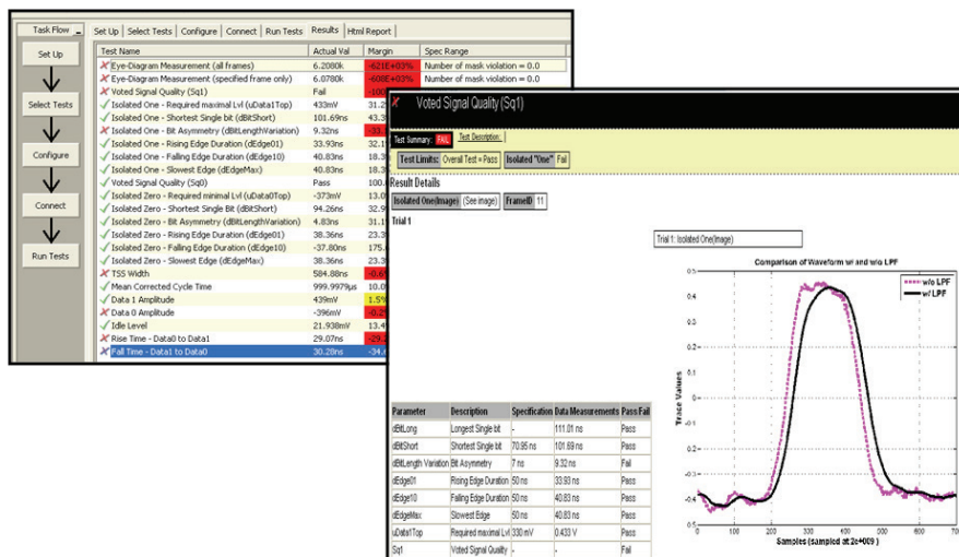
图 6. 使用 Keysight InfiniiVision X 系列示波器实施的 FlexRay 物理层一致性测试。
