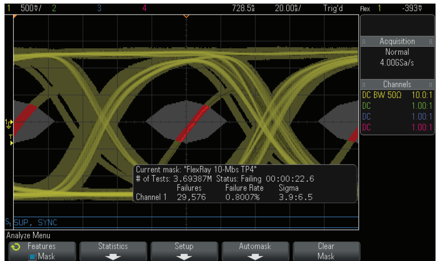
图 4. 对 FlexRay 总线的眼图模板测试显示有一个偏移比特。
