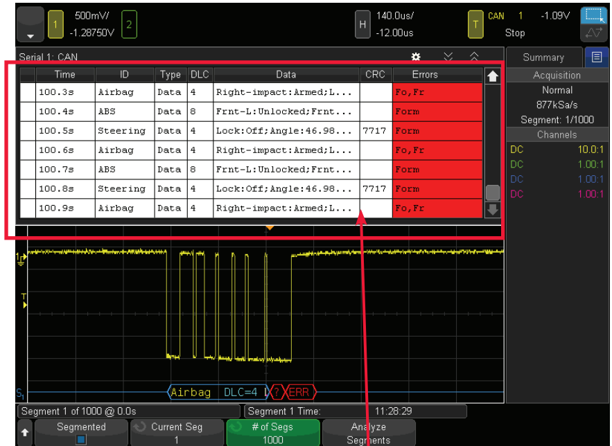
图 3. 使用分段存储器在 100 秒时间内捕获 1000 个连续的 CAN 总线误码。
