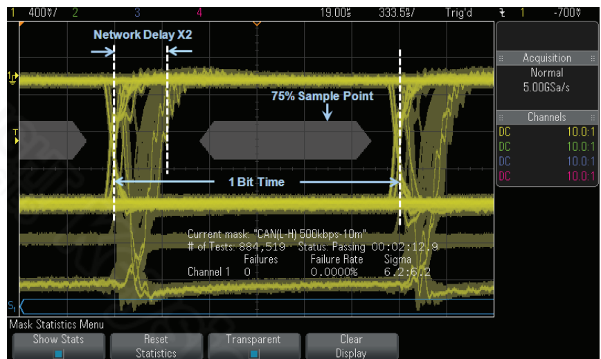
图 5. 使用 Keysight InfiniiVision X 系列示波器实施的 CAN 眼图模板测试。
