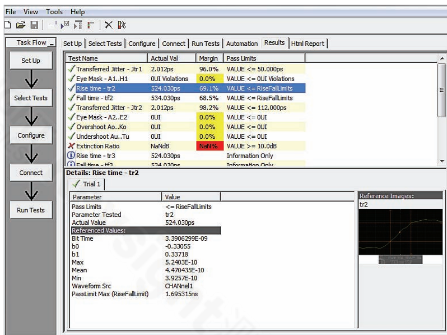
图 7. 通过使用 Keysight Infiniium S 系列示波器执行一系列自动测试得到的 MOST150 物理层一致性汇总测试报告。
