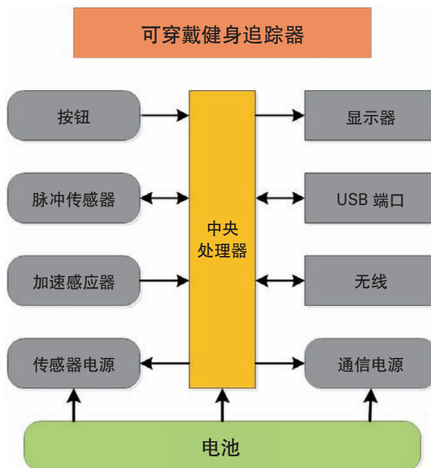
图 1. 可穿戴健身追踪器框图
